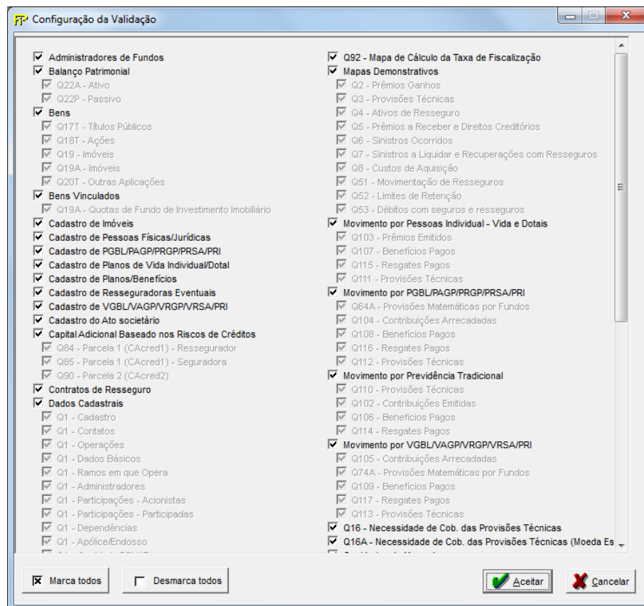
Figura 208: TFrmConfigValidacao. Configuração da validação
