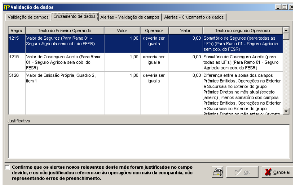
Figura 205: Tela de Validação – Cruzamento de Dados
